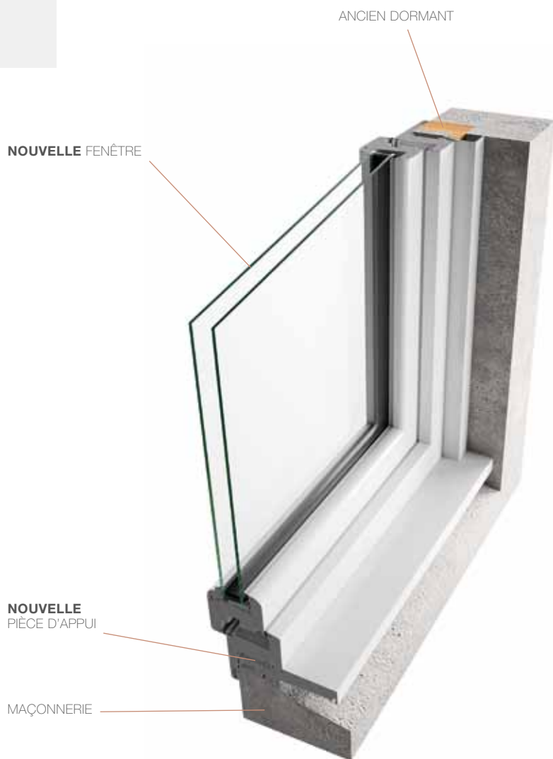
POSE EN RÉNOVATION AVEC DÉPOSE DE L'APPUI
